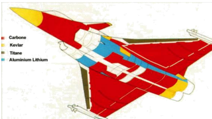
Exemple des matériaux utilisés sur un Rafale
