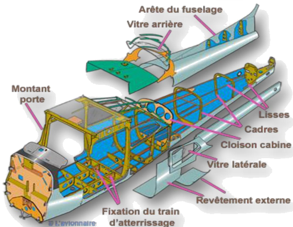
Structure Métal
